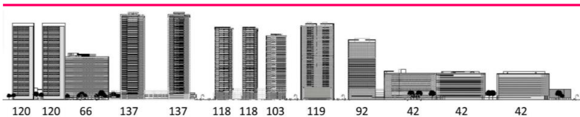
Figura 2: Fachada para a Bacia do Pina | Gabarito revisado e gabarito inicial (linha rosa). Fonte: PNR, 2015.
